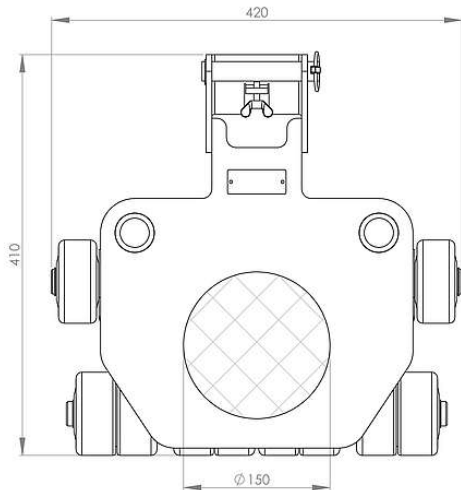
JLF 5 | Bestell-Nr. 16 050 085-D | Draufsicht JLF 5 | Order No. 16 050 085-D | Top view
