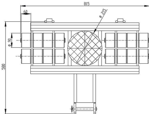
JLB 16 S Vu | Bestell-Nr. 05 161 090-V | Draufsicht JLB 16 S Vu | Order No. 05 161 090-V | Top view
