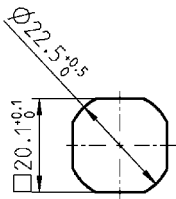
Lochbild
