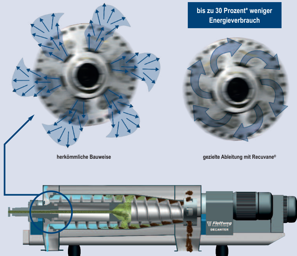
Modell: Ableitung des Zentratwassers
