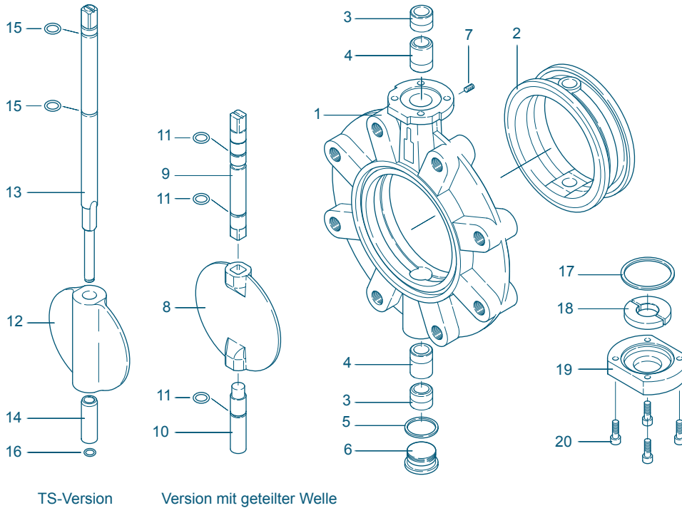
Pos. 17-20: Abschlussdeckel für Klappen ≥ da 400
