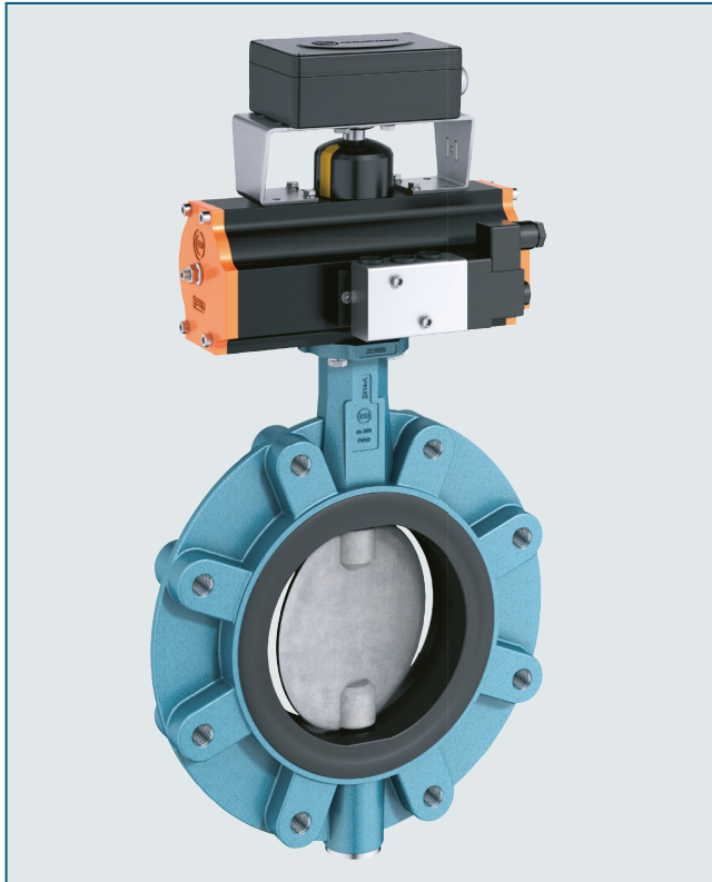
Weichdichtende, zentrische Anflanschklappe mit reduziertem Innendurchmesser für die PE/PP-Verrohrung.
