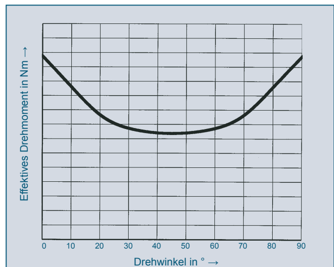
Drehmomentverlauf eines doppelwirkenden Schwenkantriebs.
