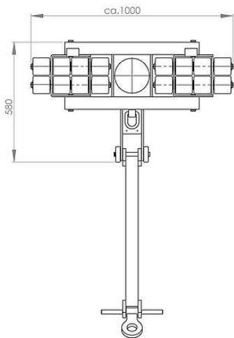
JL 14 K Vu | Bestell-Nr. 07 140 085-D | Draufsicht JL 14 K Vu | Order No. 07 140 085-D | Top view
