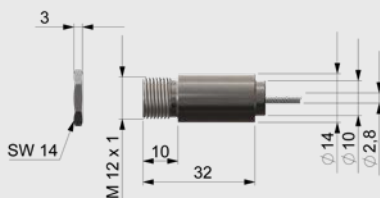
Abmessungen optris® CSmicro 3M CF1
