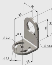
Montagewinkel, fest (ACCTFB)
