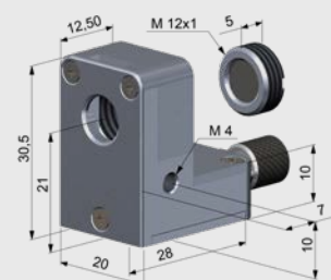
Freiblasvorsatz mit integrierter CF-Vorsatzlinse (ACCTAPLCF)
