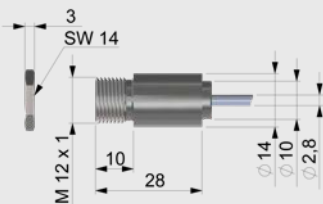
Abmessungen optris® CSmicro 3M SF/3M CF
