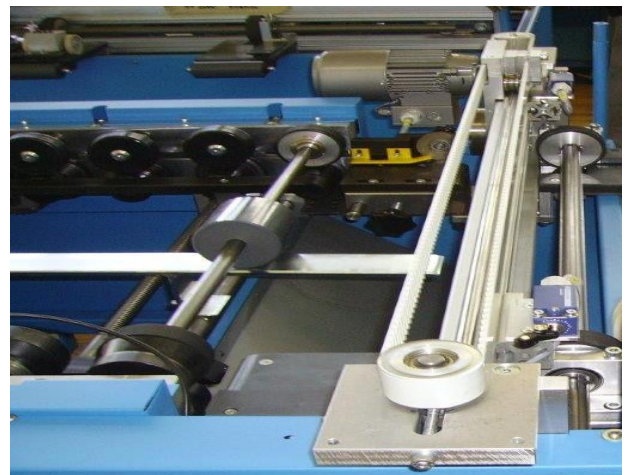
Antrieb der Schere mittels Zahnriemen (Schlupffrei)
