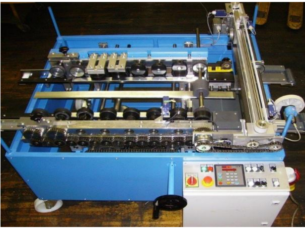
Maschine ohne Schutzhaube
