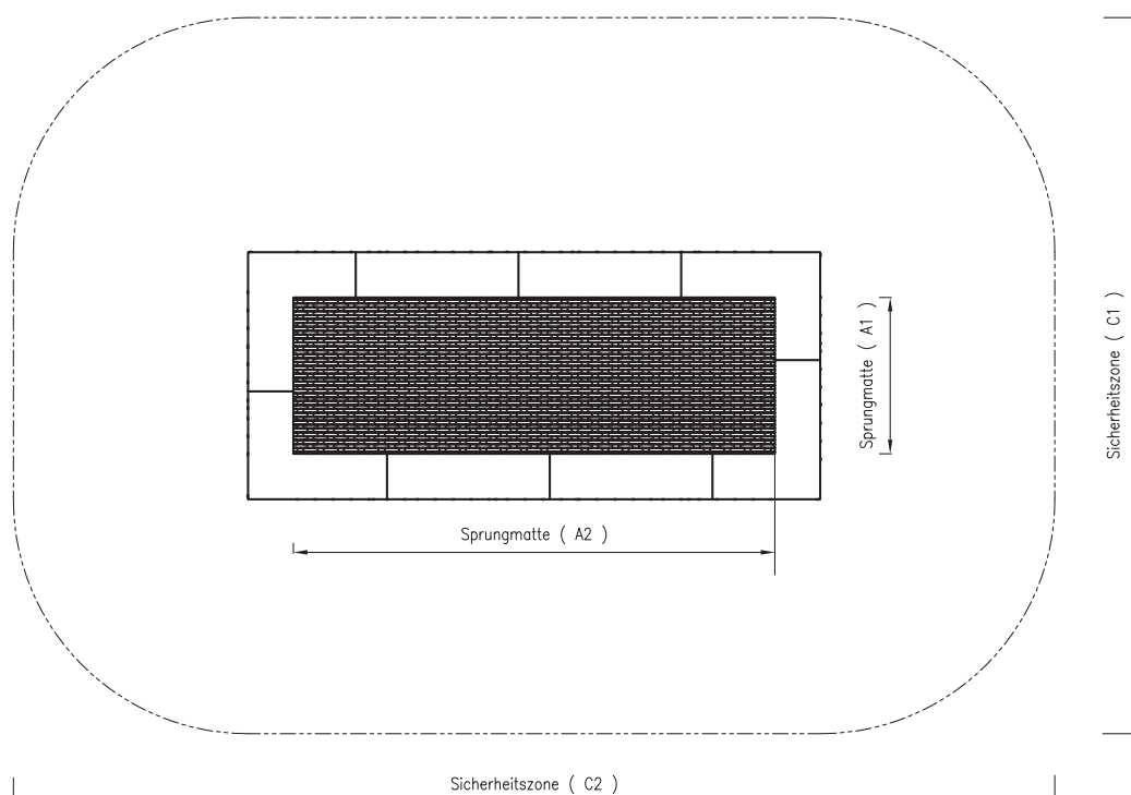
Abbildung 3: Draufsicht mit markierter Sicherheitszone.
