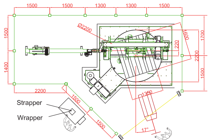
KZV-111-24 P20 mit Wickler 2.200 (Abbildung zeigt Optionen)
