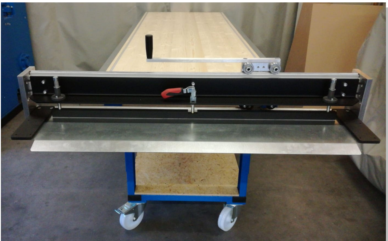
Zuschneid- und Ablängttisch optional inkl. Handschere 1000-1300mm
