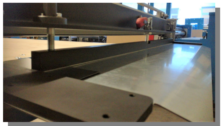
Handschere mit Niederhalter (gummiert) und Obermesser mit integrierter Führungsrolle
