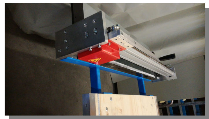
Integrierte Handschere (1000-1300mm) abklappbar, falls vorübergehend nicht benötigt
