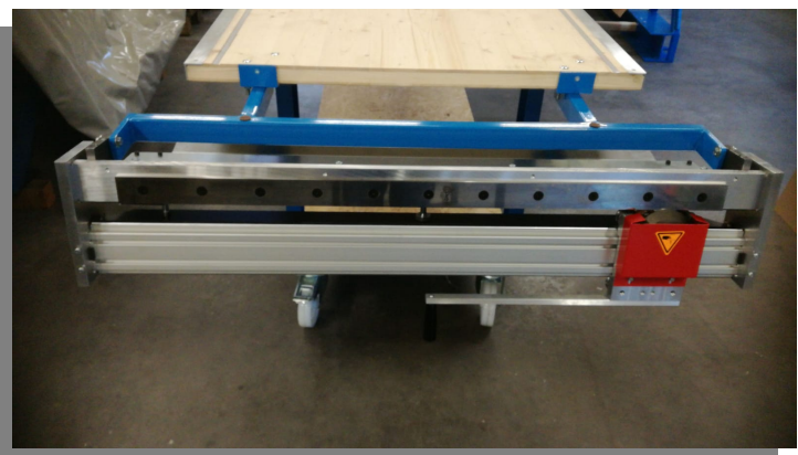
Handschere in abgeklapptem Zustand (integrierter Wendemechanismus)
