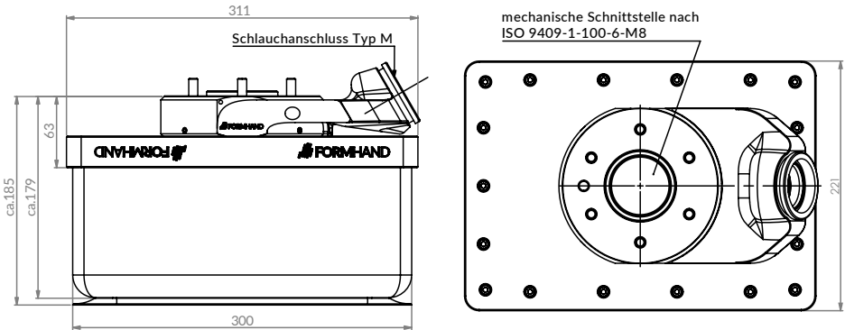
Abbildung: Ansichten des FORMHAND-Modul FH-E3020 in der Standardkonfiguration Illustration: Views of FORMHAND-Module FH-E3020 in standard configuration
