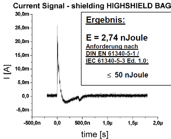
Stromsignal – ESD-Simulator mit HS-Beutel (HBM-Entladung mit 1.000 Volt)
