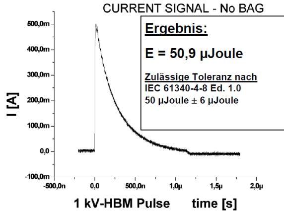
Stromsignal – ESD-Simulator ohne Verpackungsbeutel (HBM-Entladung mit 1.000 Volt)
