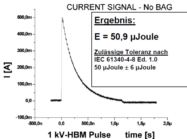
Stromsignal – ESD-Simulator ohne Verpackungsbeutel (HBM-Entladung mit 1.000 Volt)
