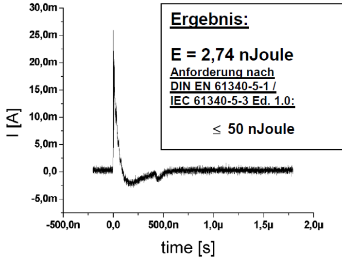
Stromsignal – ESD-Simulator mit HS-Beutel (HBM-Entladung mit 1.000 Volt)
