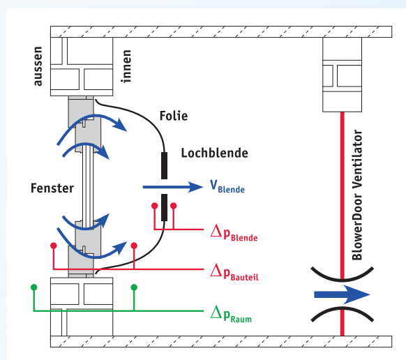
Prinzipsschnitt zur Bestimmung der Fugendurchlässigkeit von Fenstern
