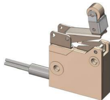
Type 7M26 : Simple Lever - Direct Action -
